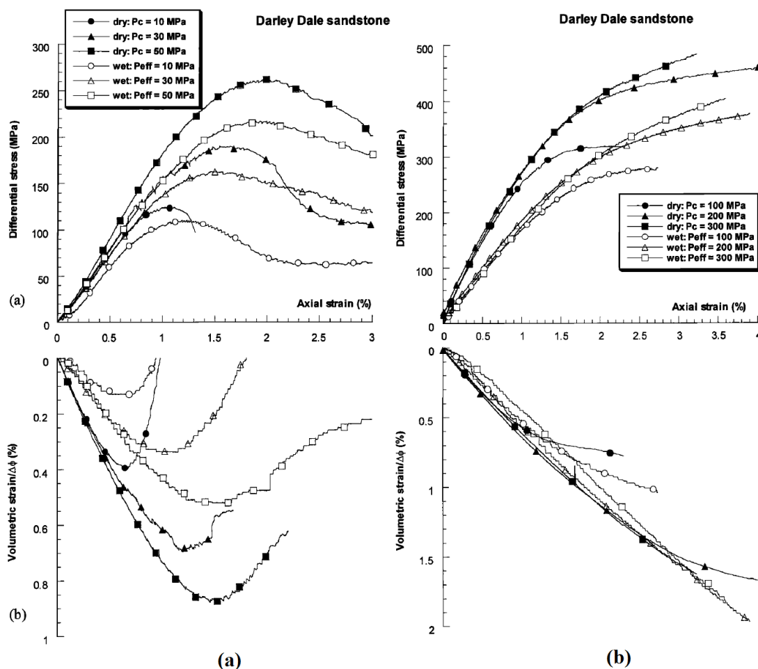
FIGURE 1.15 – Essais triaxiaux à différentes pressions de confinement sur des échantillons saturés et secs en grès de Darley Dale ; symboles vides : échantillons saturés ; symboles remplis : échantillons secs [8]. (a) Essais à faibles confinements et (b) Essais à forts confinements : déformation axiale en fonction de la contrainte déviatoire (en haut) et déformation volumique (en bas).
